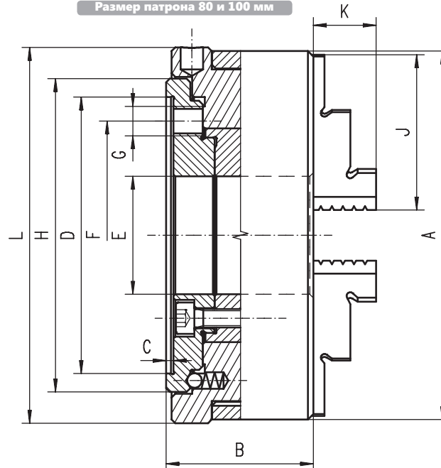
Размер патрона 80 и 100 мм
