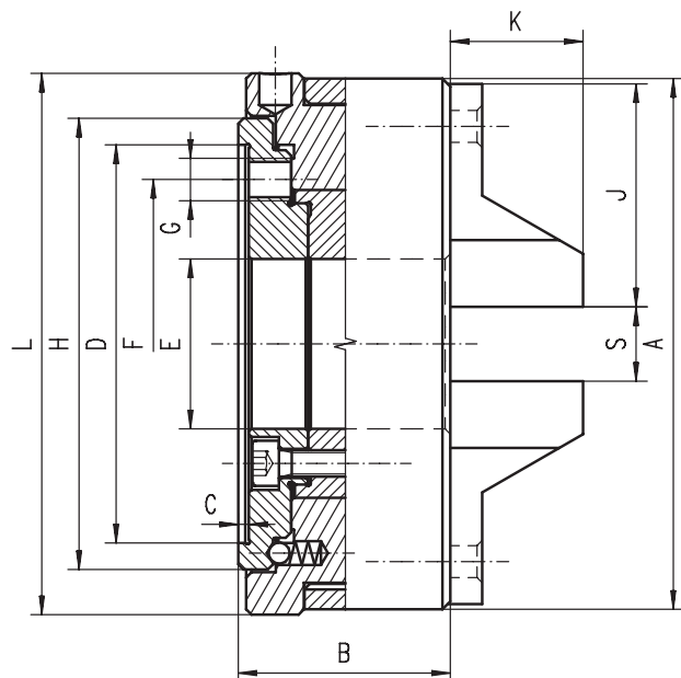
Размер патрона 80 and 100 мм
