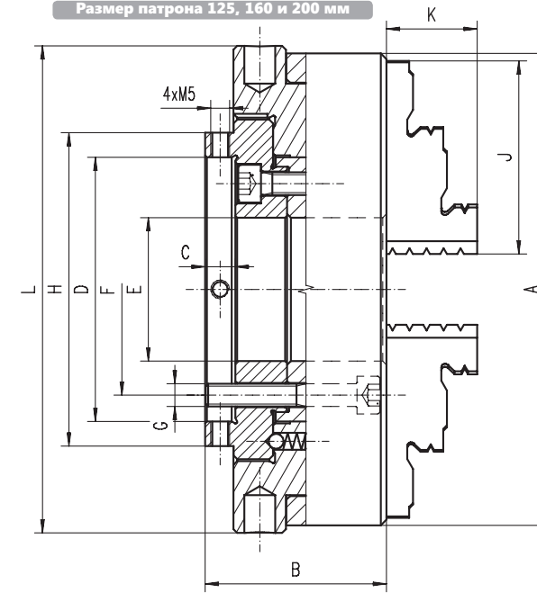
Размер патрона 125, 160 и 200 мм
