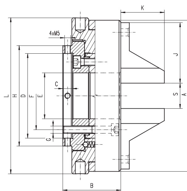
Размер патрона 125 and 160 мм
