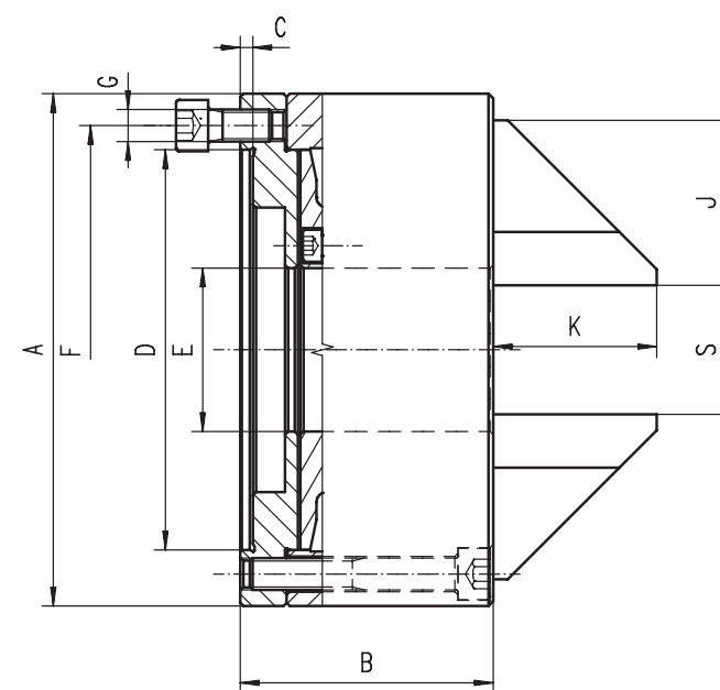
Размер патрона 160 мм
